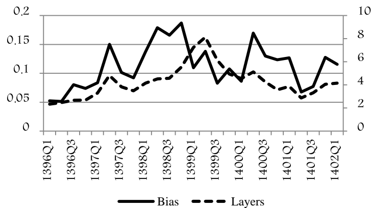
نمودار ۲. میانگین مقدار اربب PIN و تعداد لایه‌های شناسایی شده در MPIN
