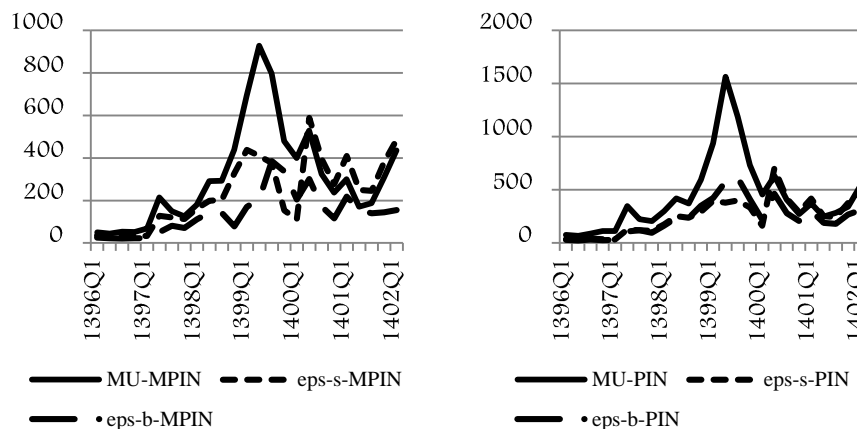
نمودار ۴. متوسط پارامترهای شدت برآورد شده در مدل MPIN و PIN
