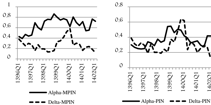
نمودار ۳. متوسط پارامترهای احتمال در مدل MPIN و PIN
